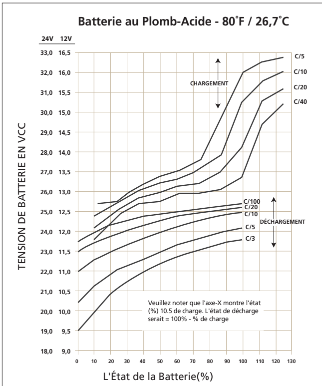
Figure. 7.1: Les courbes de charge / décharge pour 12V et 24V batterie plomb-acide
