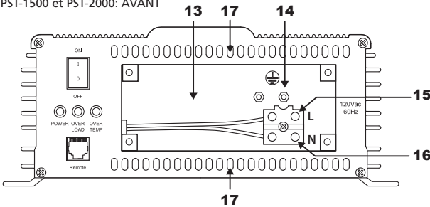
PST-1500 et PST-2000: AVANT - montrant les bornes de sortie du compartiment contenant AC pour câbler
