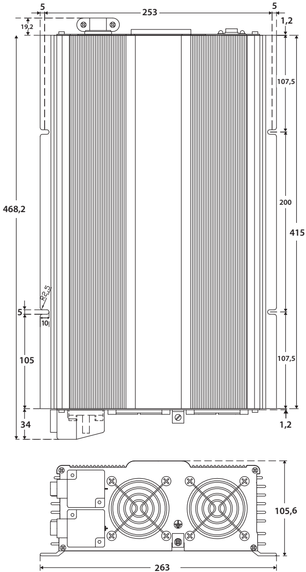
Fig. 8.1: Les Dimensions Générales et Rainures de Montages des PST-1500 et PST-2000 (NB: Dimensions en mm)
