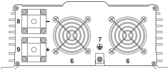
PST-1500 and PST-2000: LA DERRIÈRE
