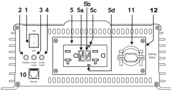
PST-1500 et PST-2000: AVANT
